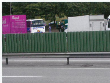
Durchstiegsbarriere für Fußgänger auf Autobahnen und Schnellstraßen Passage barrier for pedestrians on highways
